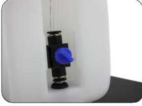
Püskürtme hacmini ayarlayabilen vana sistemi
